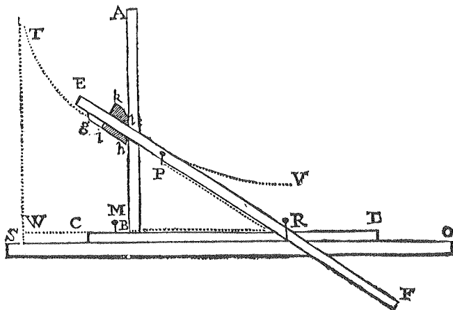
Plaat 9. John Perks' sleepinstrument voor de hyperbool- quadratuur (zie noot 15).
